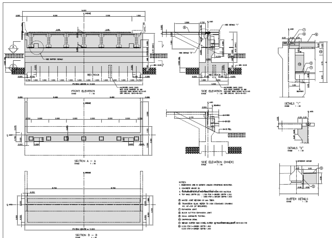
รูปที่ 6-9 รูปตัดช่วงตอม่อตับริม (ต่อ)
