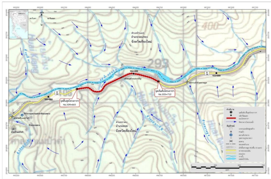
รูปที่ 5-12 ทิศทางการไหลของการระบายน้ำในพื้นที่โครงการ
