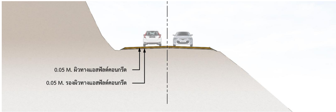
รูปที่ 6-14 รูปแบบโครงสร้างชั้นทาง (ปรับปรุงผิวจราจรเดิม)
