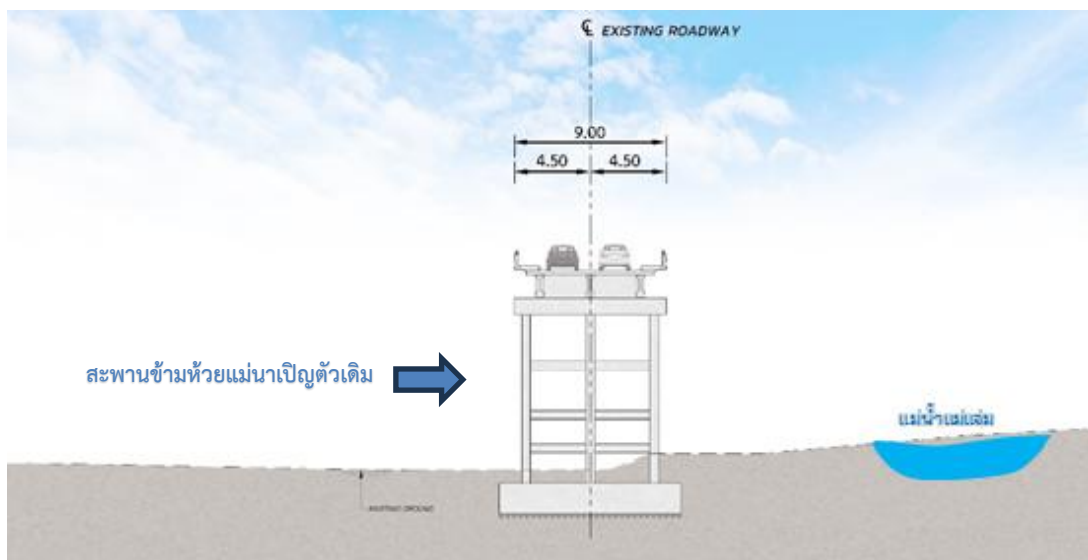
รูปที่ 5-6 รูปตัดโครงสร้างสะพานข้ามห้วยแม่น้ำเปิงตัวเดิม
