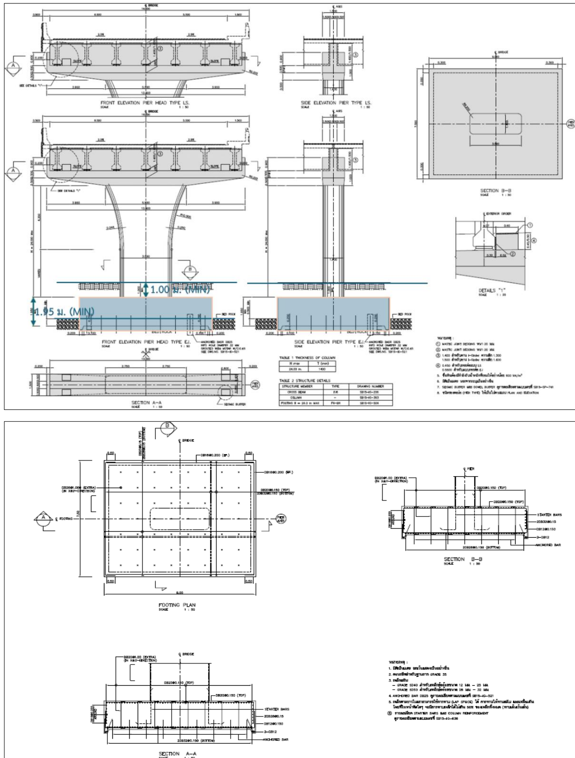
รูปที่ 6-11 งานออกแบบฐานรากสะพาน
