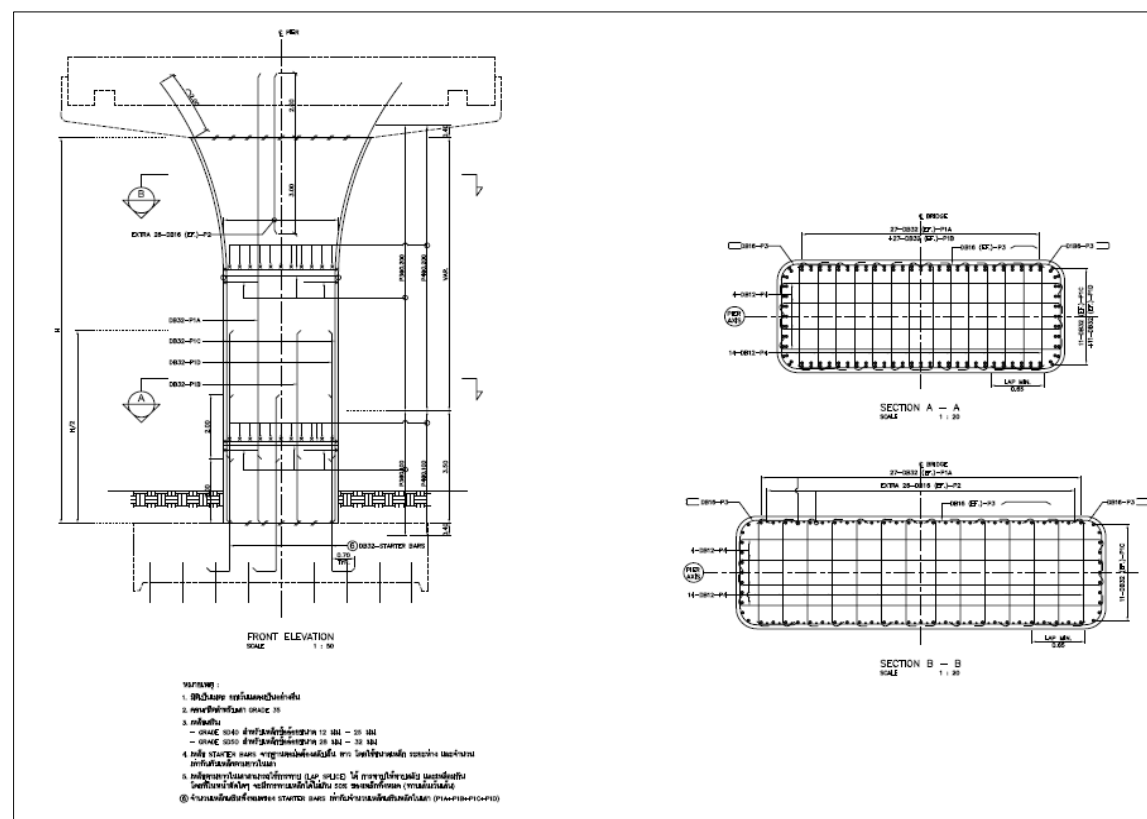
รูปที่ 6-11 รูปตัดช่วงตอม่อกลาง (ต่อ)
