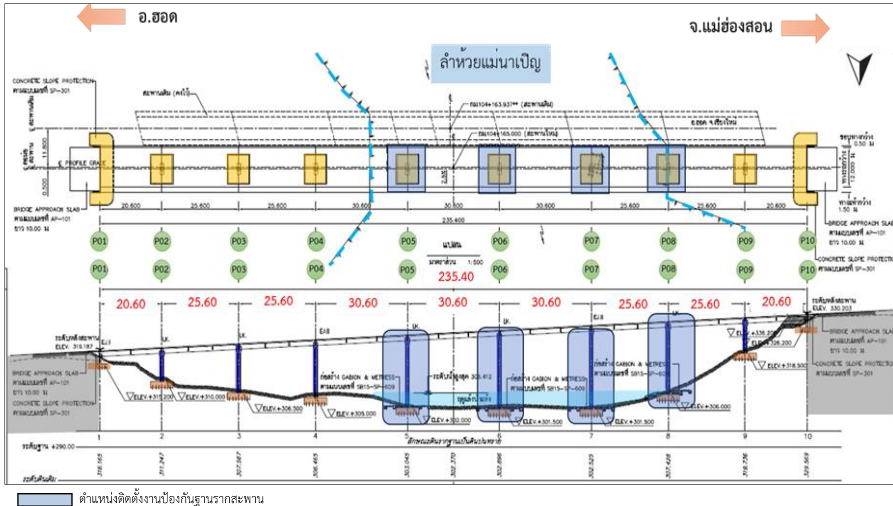
รูปที่ 6-13 ตำแหน่งติดตั้งงานป้องกันฐานรากสะพาน
