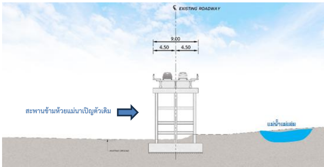
รูปที่ 5-5 รูปตัดโครงสร้างสะพานข้ามห้วยแม่น้ำเปียงตัวเดิม
