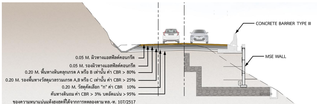
รูปที่ 6-16 รูปแบบโครงสร้างชั้นทาง (ขยายพื้นที่ผิวจราจรที่เป็นคันทางใหม่)
