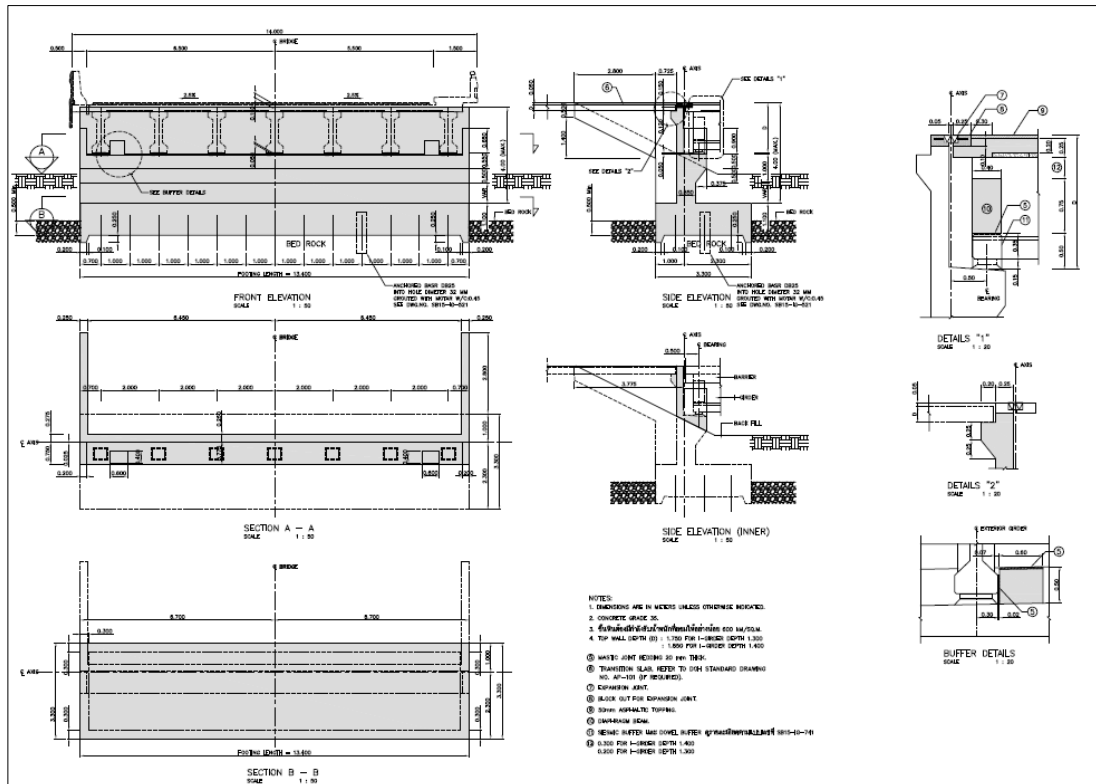
รูปที่ 6-10 รูปตัดช่วงตอม่อตบริม (ต่อ)
