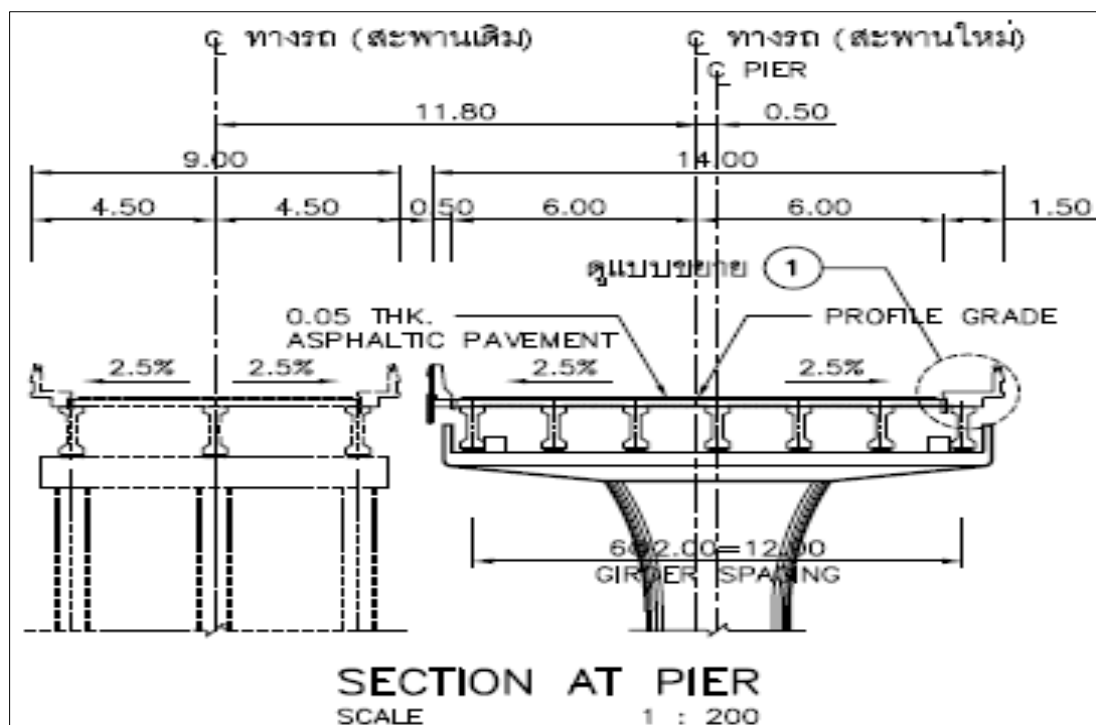
รูปที่ 6-11 รูปตัดช่วงตอม่อกลาง
