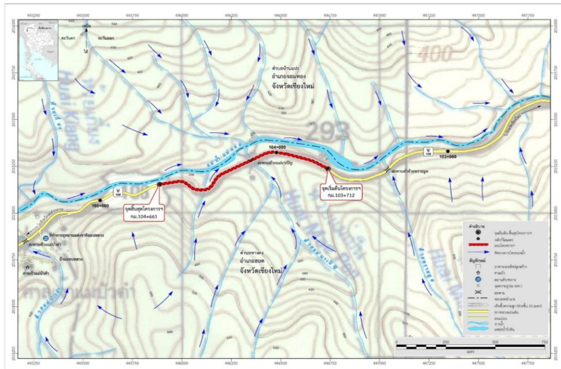
รูปที่ 5-11 ทิศทางการไหลของการระบายน้ำในพื้นที่โครงการ
