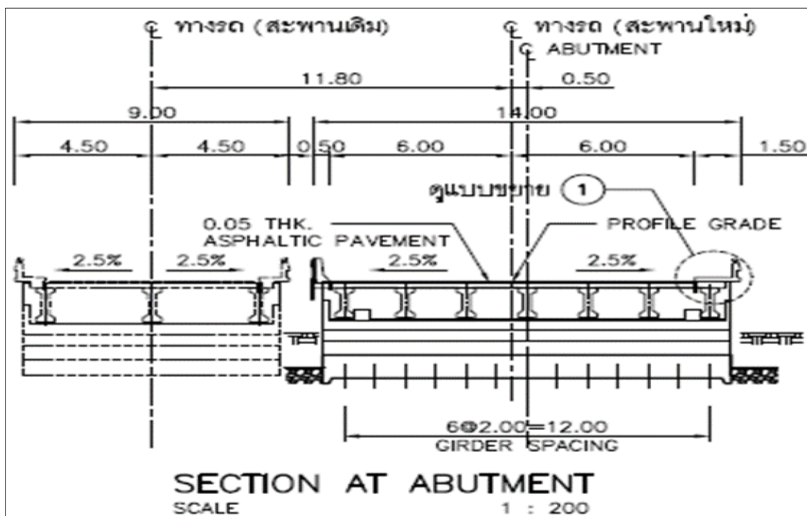
รูปที่ 6-10 รูปตัดช่วงตอม่อตบริม
