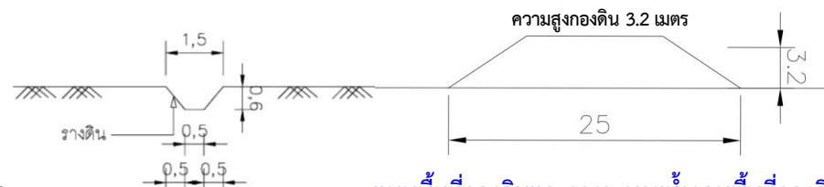
แบบพื้นที่กองดินและรางระบายน้ำรอบพื้นที่กองดิน
