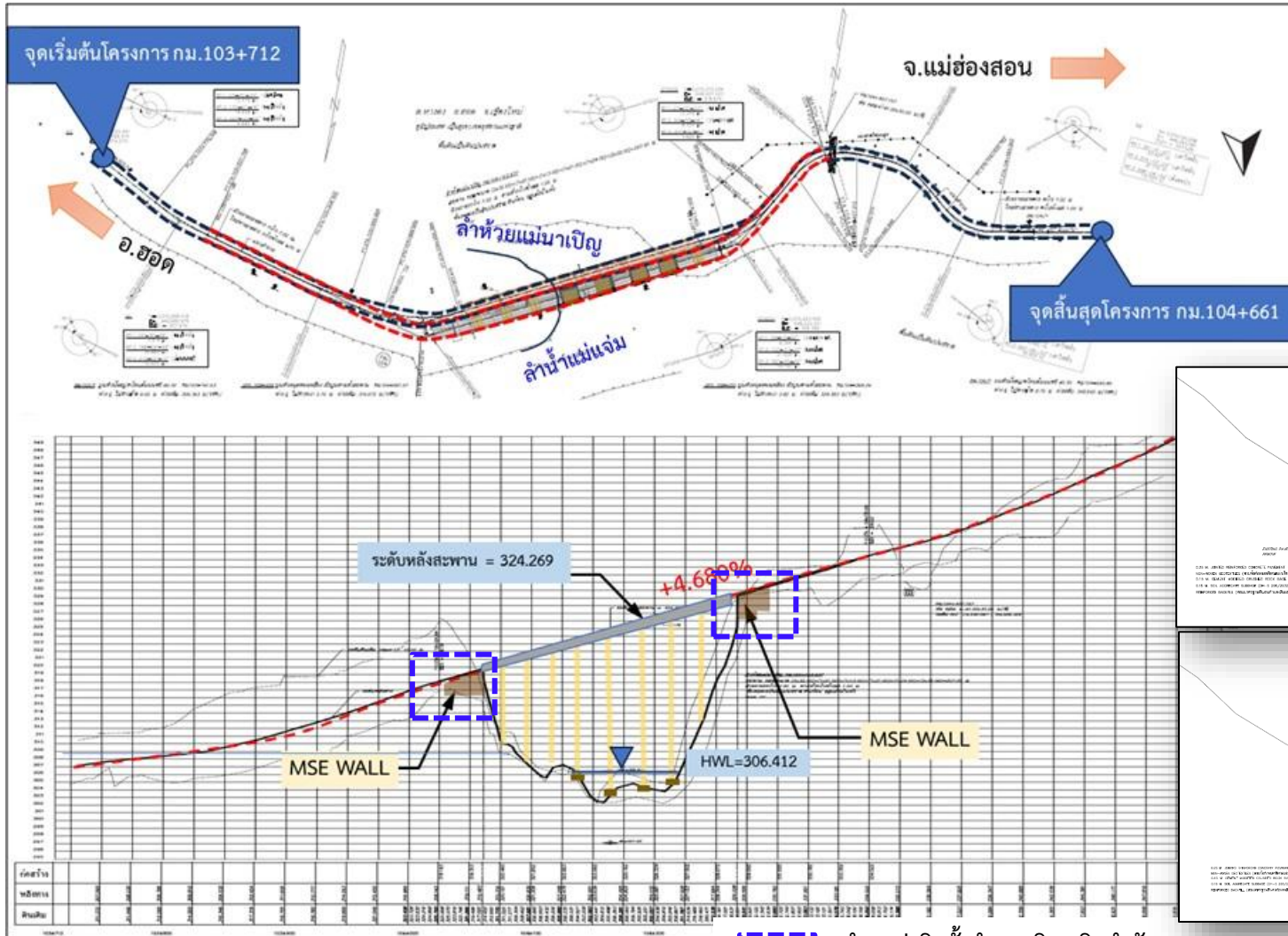
ตำแหน่งติดตั้งกำแพงดินเสริมกำลัง (Mechanically Stabilized Earth Wall)
